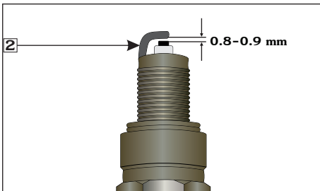
(2) Electrodo lateral
