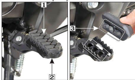
(1) Gomas (2) Posapiés del conductor (3) Proyecciones
