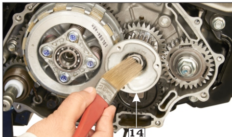
(14) Filtro centrífugo
