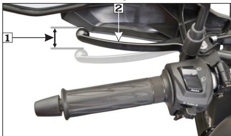
(1) Juego libre: 10-20 mm (2) Palanca
